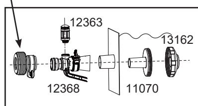
Adaptateur fileté B
