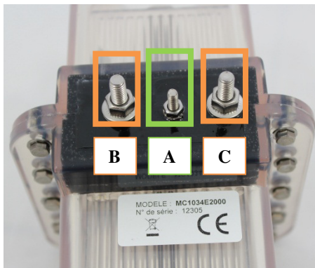
B Raccordement électrique de la cellule A raccorder indifféremment aux fils bleu et marron C
