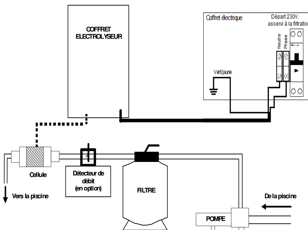
POSITION POSSIBLE DE LA CELLULE
